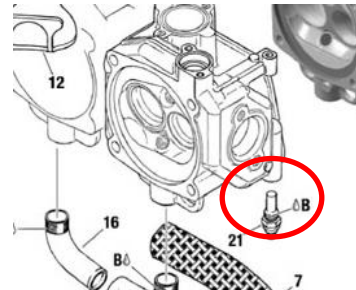
●ROTAX 912 純正センサー (エンジンに付属しています。) #02-965-531 ..... ¥25,390 (10×1.5mm thread)
